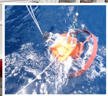
▲研究で使用している音の送受波器
